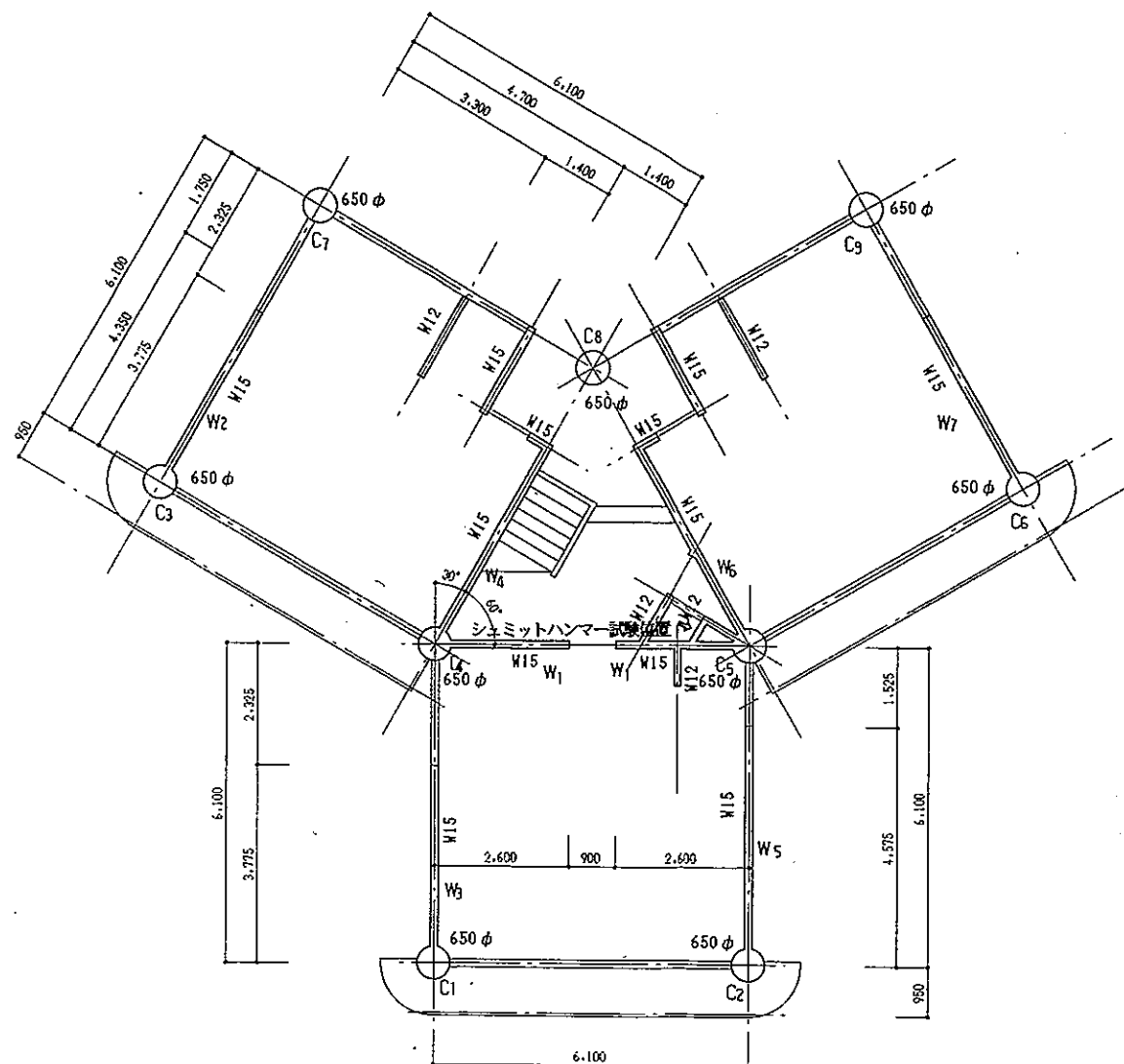
1 階 平 面 図
