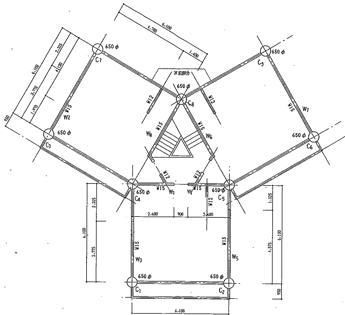
2階・3階・4階平面図
