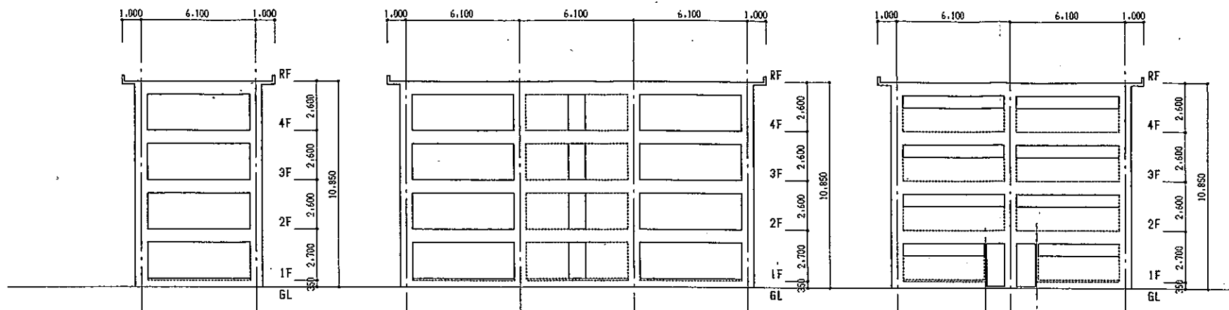
軸 組 図
