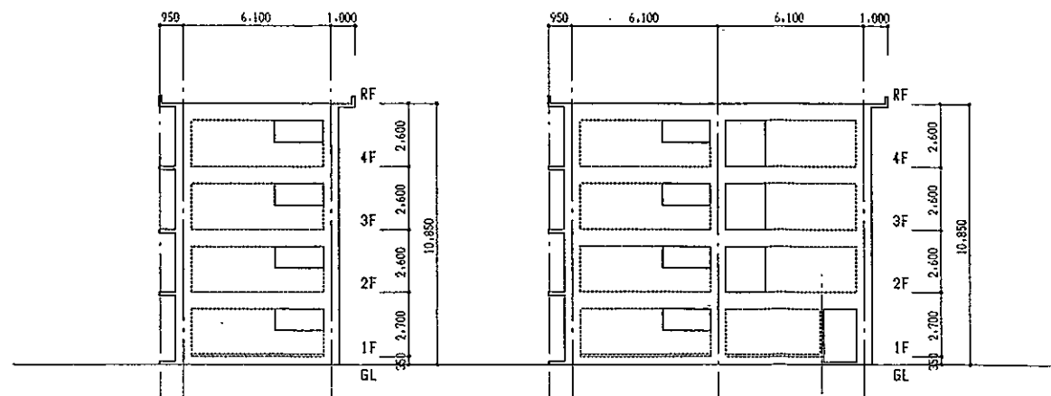
軸 組 図
