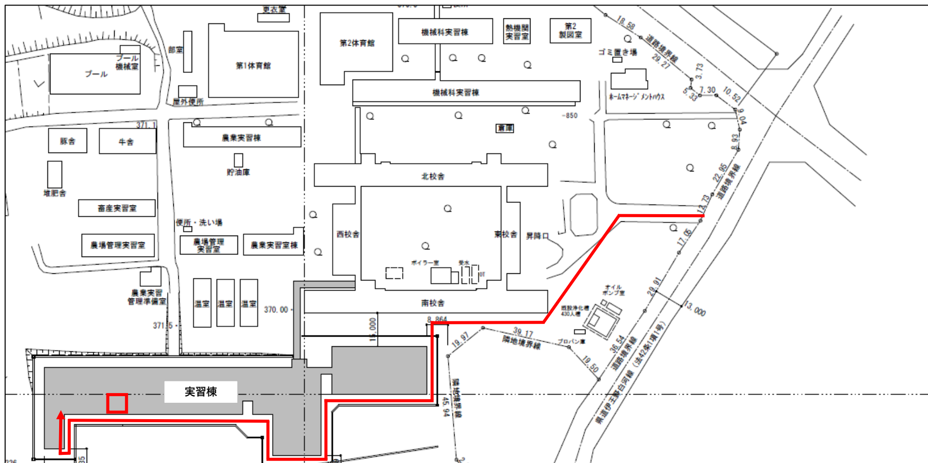
福島県立白河実業高等学校 校舎等配置図
