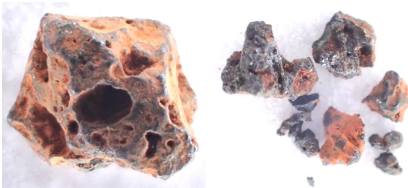
燃料デブリサンプルの外観・拡大写真（真上から撮影）
