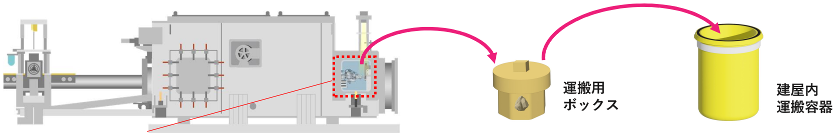
エンクロージャ側面ハッチから「運搬用ボックス」を取り出す様子
