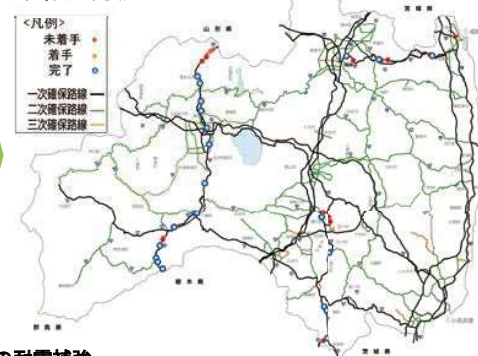
道路橋梁の耐震補強
