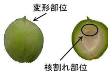
図2 核頂部の障害と果頂部の変形
