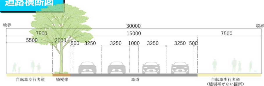
標準横断面図(現状)
