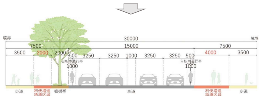
標準横断面図(利便増進誘導区域指定後)
