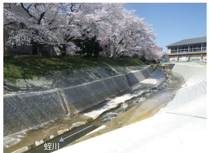
蛭川（福島市瀬上町） 開削護岸
