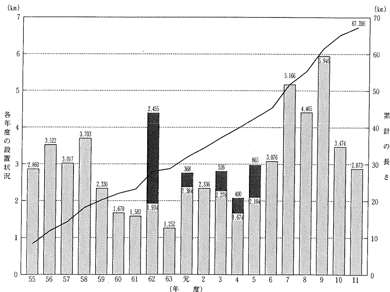
図－23 県内の高速自動車道に係る遮音壁の設置状況
