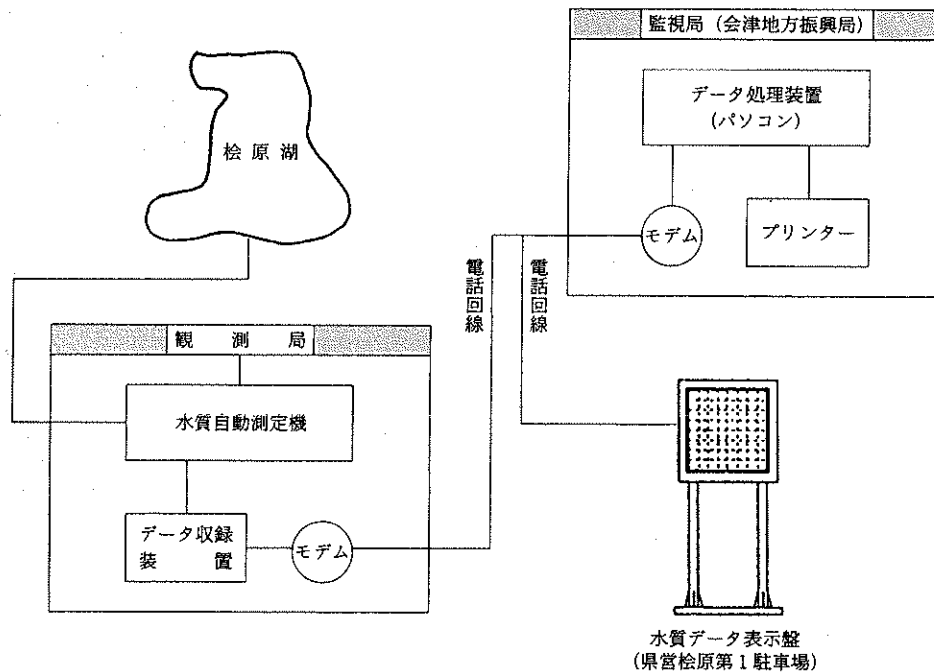
図-18 水質自動モニタリングシステムの系統図
