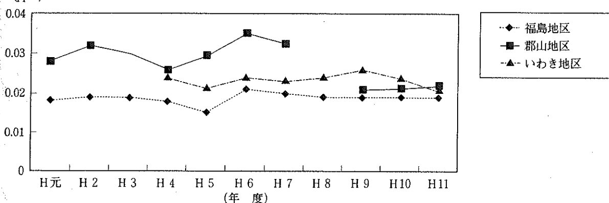
図-6 二酸化窒素濃度（年平均値）の経年変化 (ppm)
