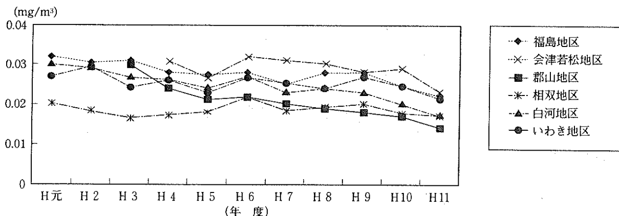
図-4 浮遊粒子状物質濃度（年平均値）の経年変化
