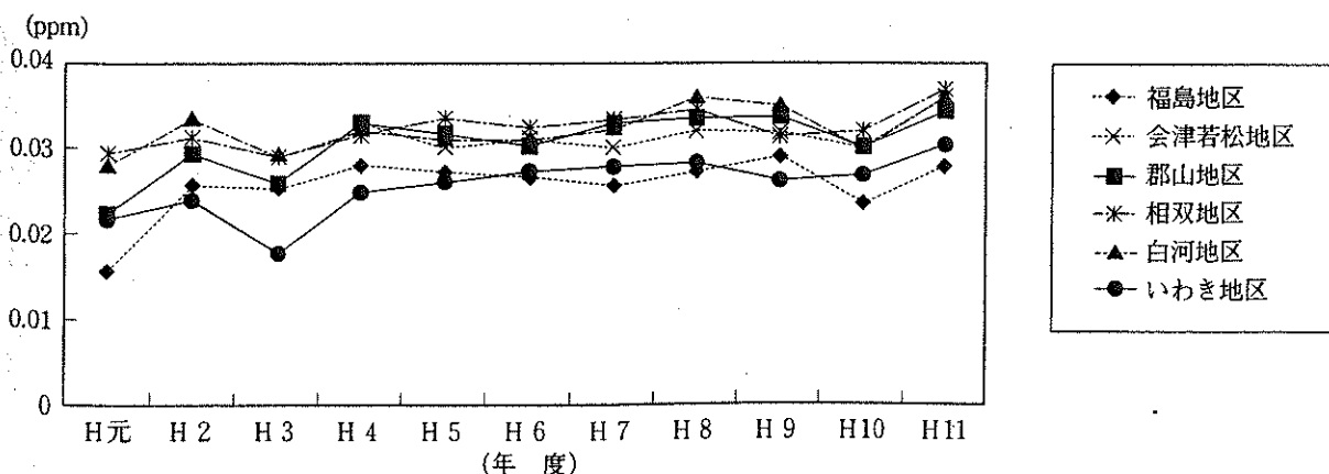
図-3 光化学オキシダント濃度(夜間の年平均値)の経年変化
