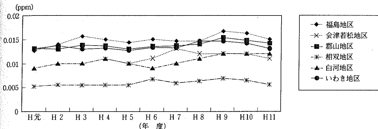
図-2 二酸化窒素濃度(年平均値)の経年変化
