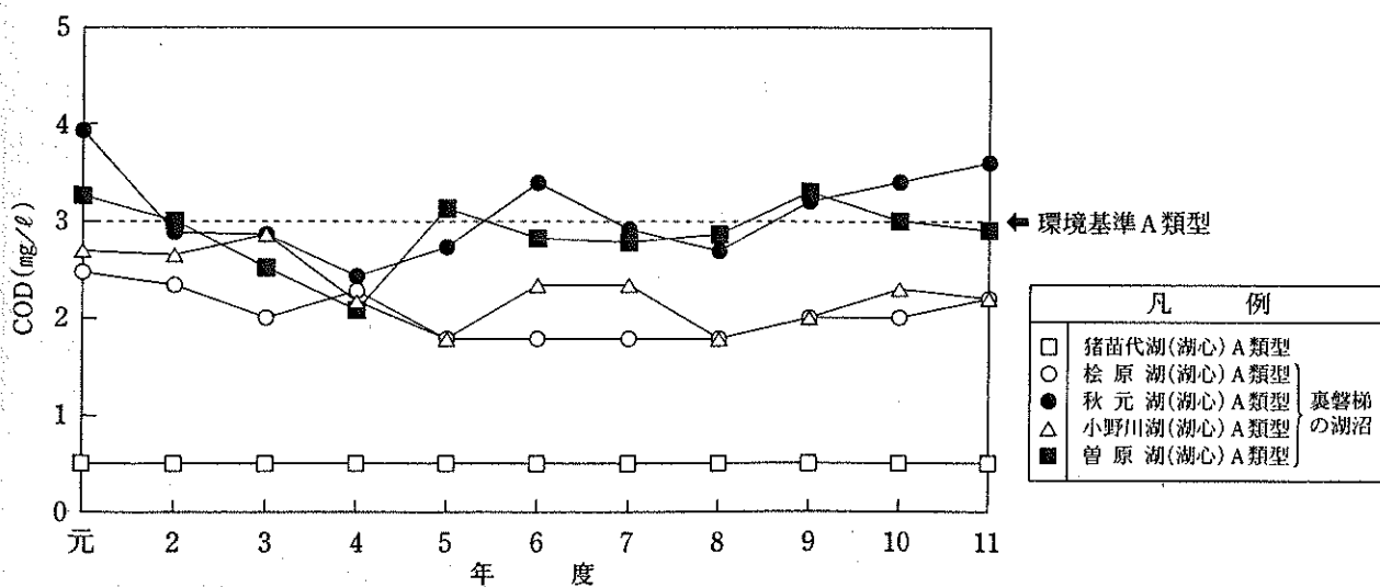
図-10 湖沼の水質 (COD 75%値) の経年変化
