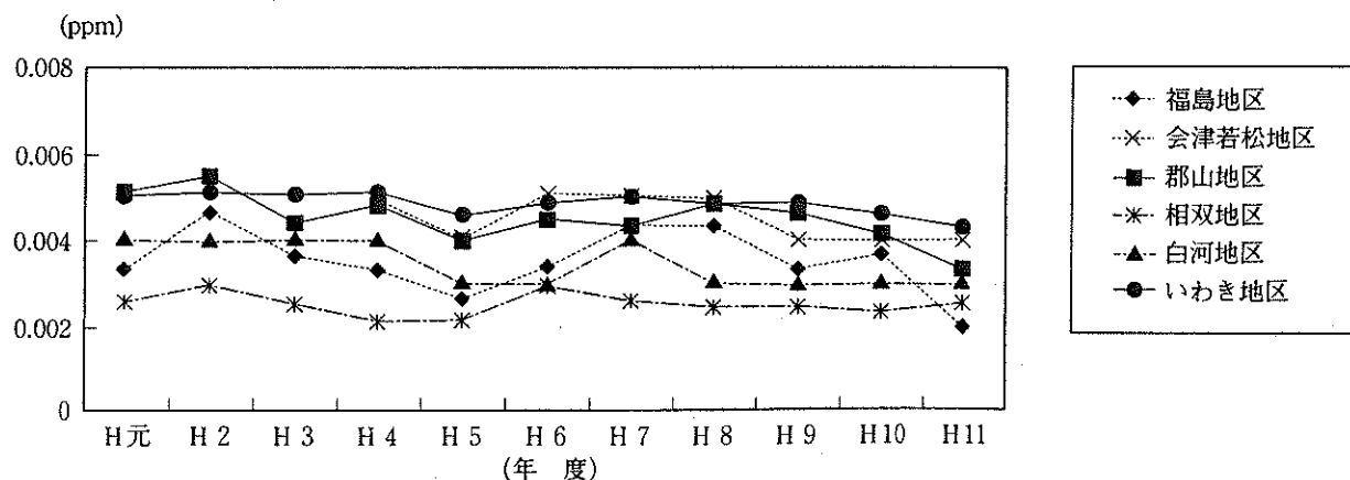
図－１ 二酸化硫黄濃度（年平均値）の経年変化
