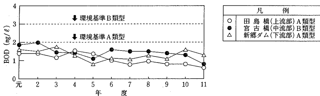
図-9 河川の水質（BOD 75%値）の経年変化
