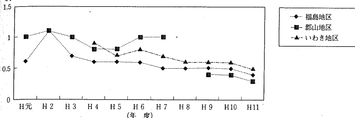
図-5 一酸化炭素濃度（年平均値）の経年変化 (ppm)
