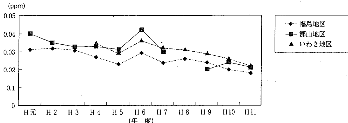
図一 7 浮遊粒子状物質濃度（年平均値）の経年変化
