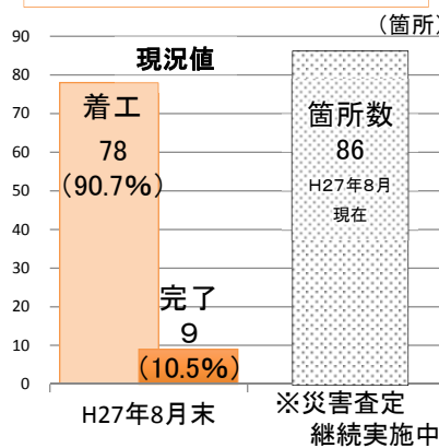
海岸施設(堤防等)の復旧状況
